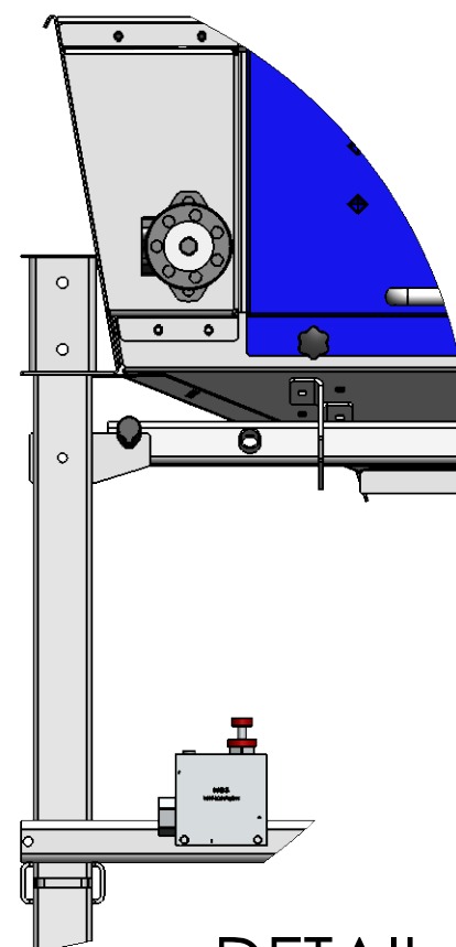
DETAIL E MAßSTAB 1 : 10
