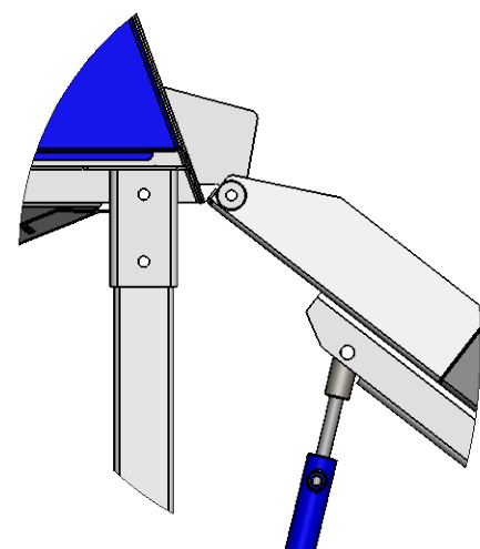
DETAIL F MAßSTAB 1 : 10
