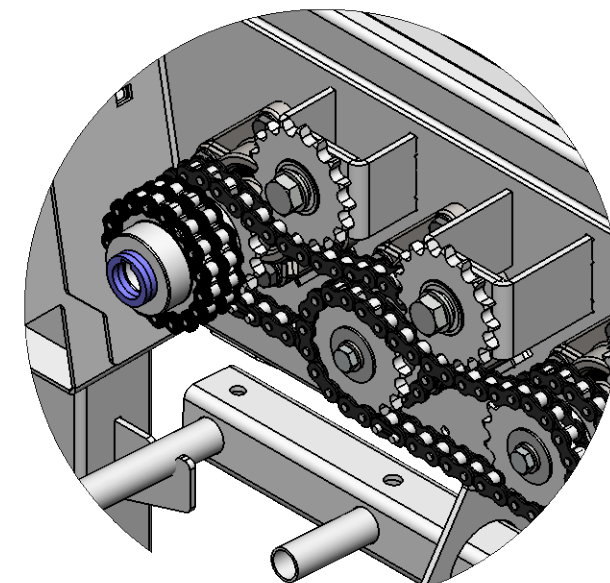
DETAIL G MAßSTAB 1 : 5
